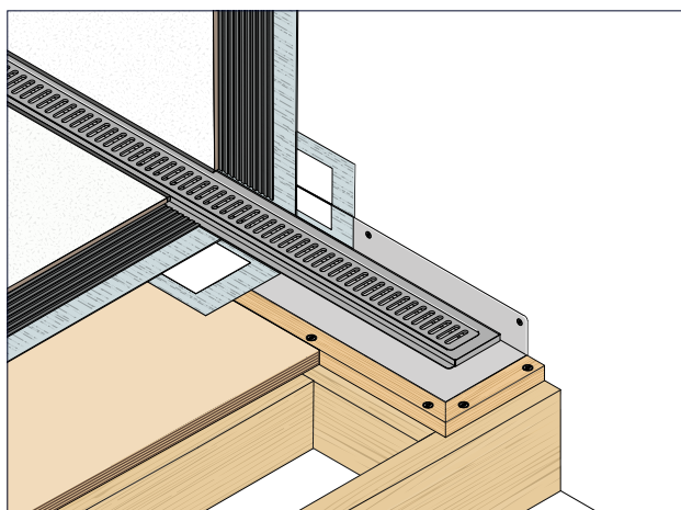
Unidrain afløb med ClassicLine ramme/rist og Montagesæt 22 mm | væg
