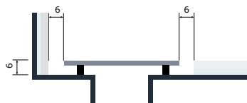
Tværsnit af afløbsarmatur uden ramme/ med Panel i børstet stål.
