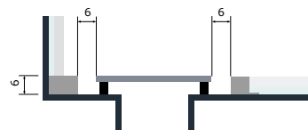
Tværsnit af afløbsarmatur med ramme/ med Panel i børstet stål.
