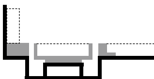
Tværsnit af afløbsarmatur med ramme / Cassette i børstet stål.
